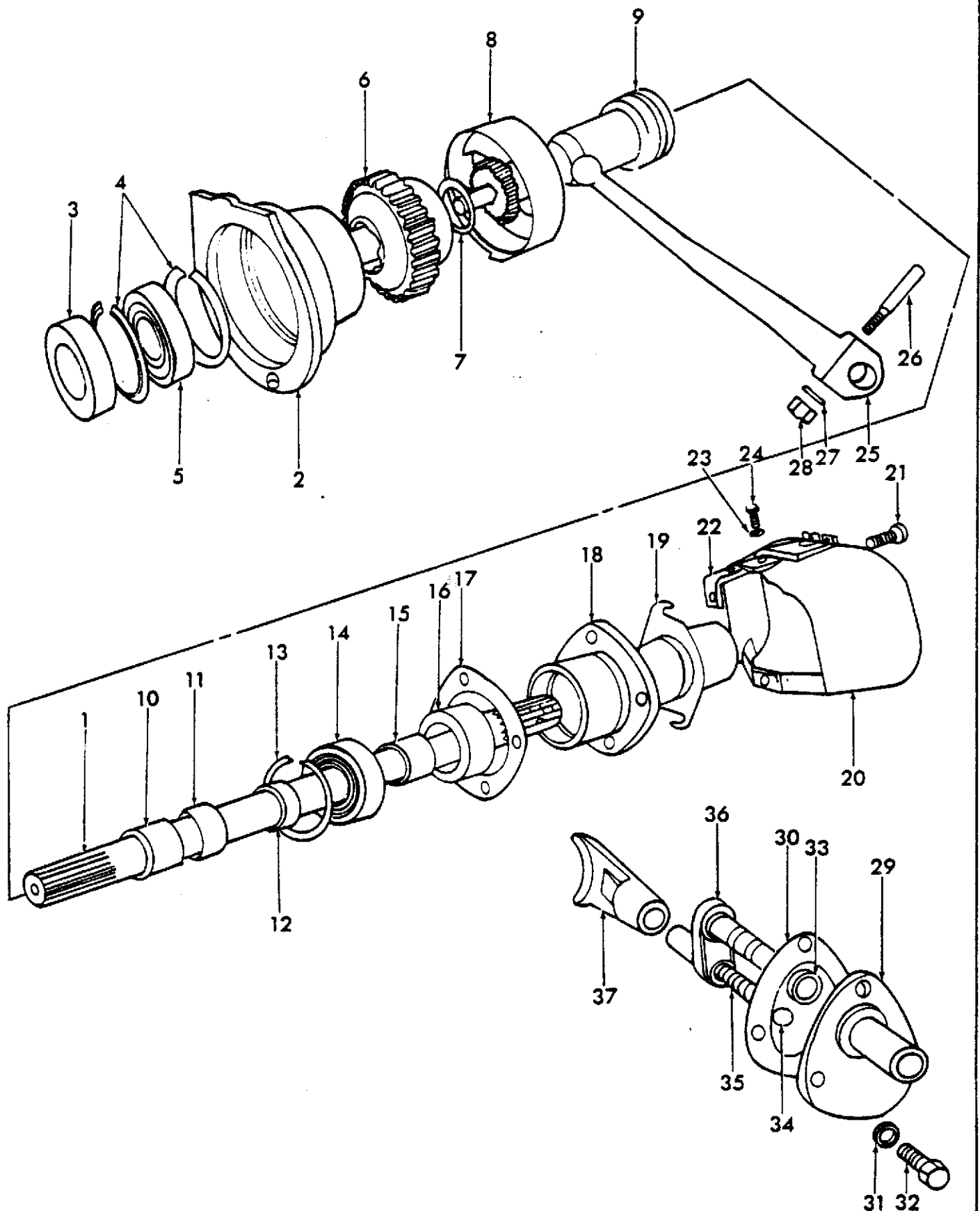
Fig. 29 Standard P.T.O.
