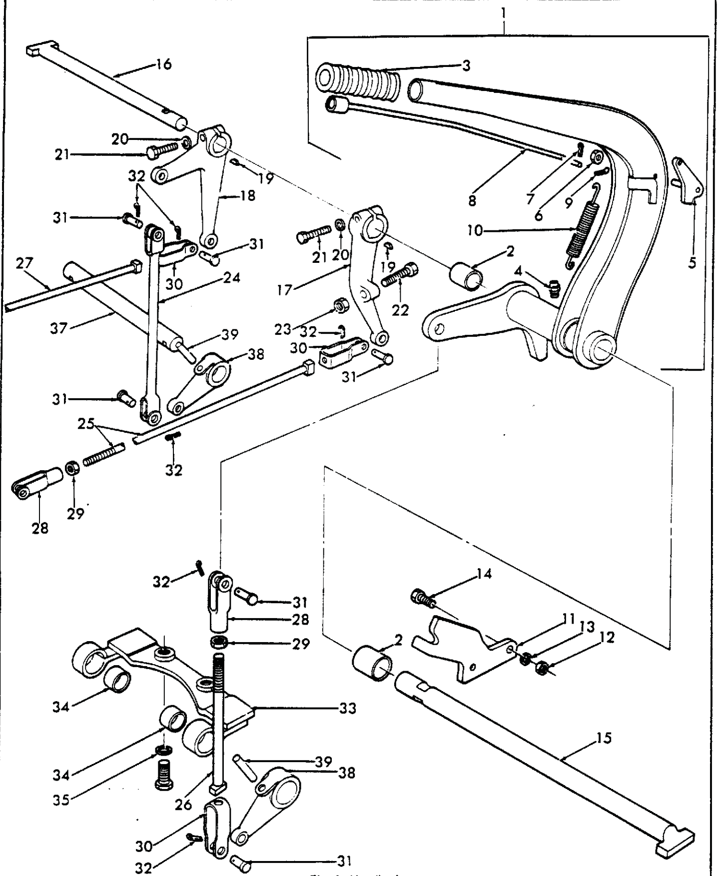
Fig. 4 Handbrake
